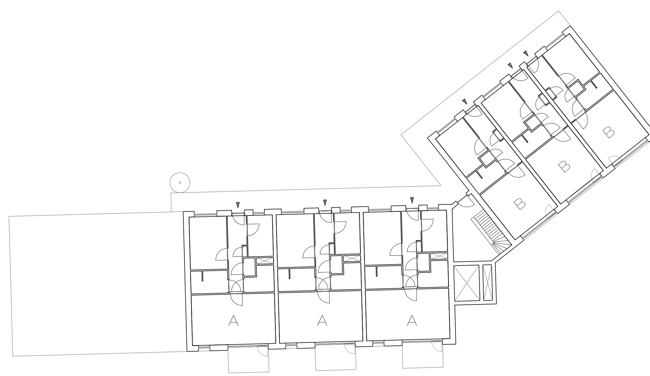
OVERZICHTS PLATTEGROND 2e verdieping
