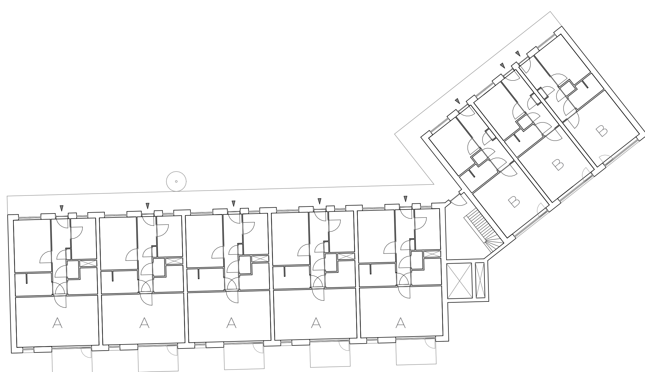
OVERZICHTS PLATTEGROND 1e verdieping
